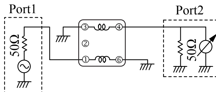
貼片共模電感器 (TCB4F - 617DB) 測試電路
