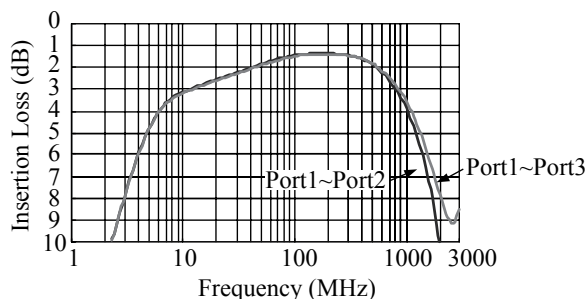
TCB4F-617PT-1667 (Impedance Ratio=50Ω:200Ω)
