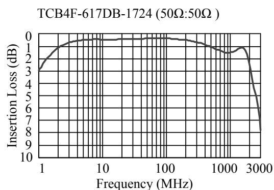
貼片共模電感器 (TCB4F - 617DB) 代表特性圖
