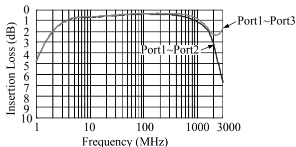
貼片共模電感器 (TCB4F - 617DB) 代表特性圖
