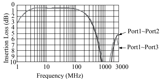
TCB4F-617PT-1664 (Impedance Ratio=50Ω:200Ω)
