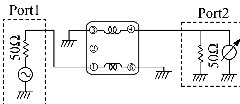
貼片共模電感器 (TCB4F - 617DB) 測試電路
