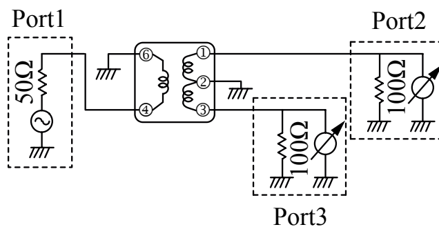
貼片共模電感器 (TCB4F - 617PT) 測試電路c
