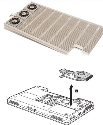
Custom Fin and Fan Assemblies
