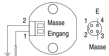
Klemmenbelegung M12 Stecker
