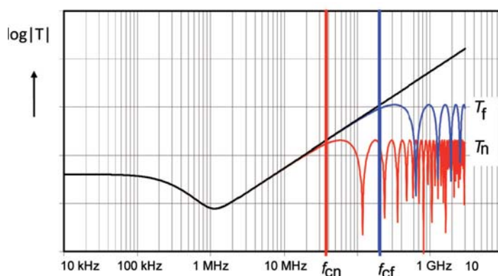
Bild 2: Gerechnete Kopplungsübertragungsfunktion T_{n,f} eines Geflechtsschirms
