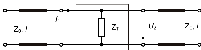
Bild 17: Messen von EMV-Dichtungen und Durchführungen, Ersatzschaltbild
