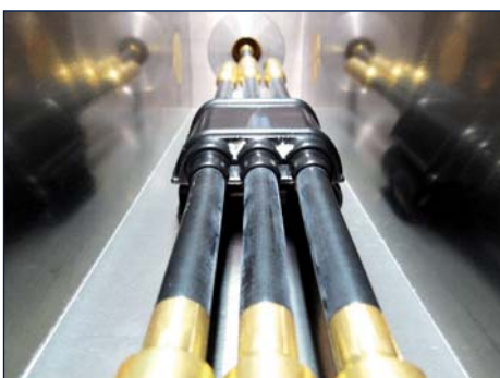
Bild 13: BK-Abzweiger in Triaxialer Zelle
