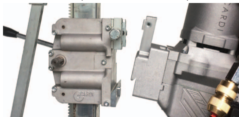
Sistema di attacco rapido a coda di rondine CARDI 306 e CARDI 400
