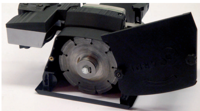
Dettaglio carter protezione dischi
