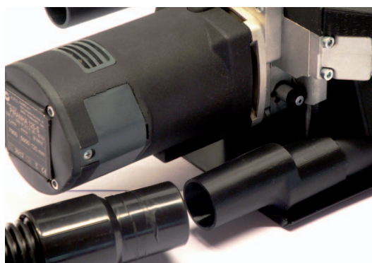
Attacco aspiratore polveri
