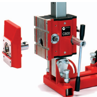
sistema di attacco rapido CAM-LOCK CARDI 606 - 805 - 1005
