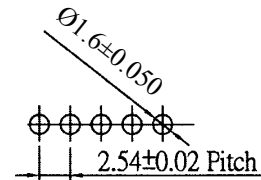
P.C.Board Layout
