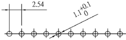
P.C.Board Layout
