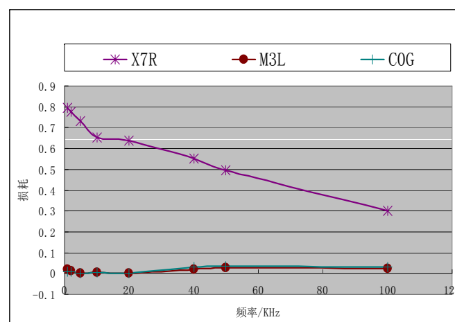
损耗-频率特性曲线
