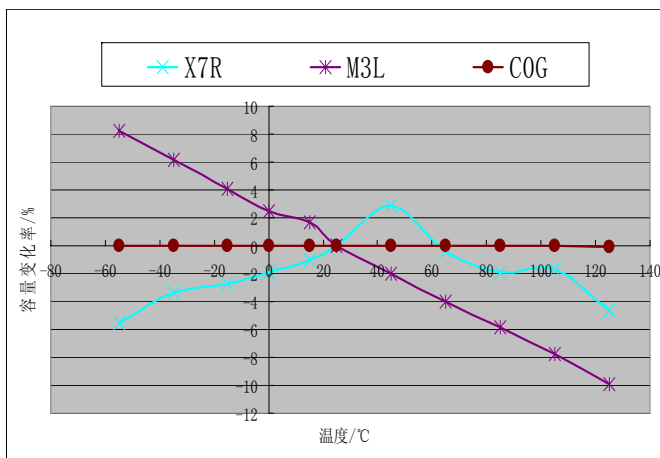
容量-温度特性曲线
