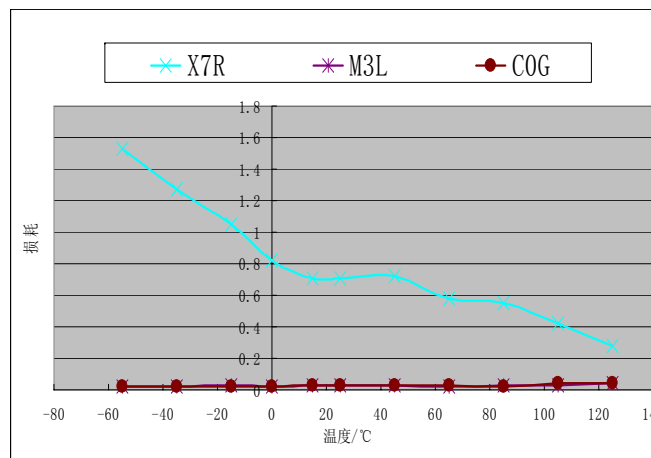
损耗-温度特性曲线
