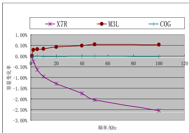
容量-频率特性曲线
