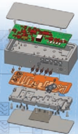
X-Band SDLVA module.
