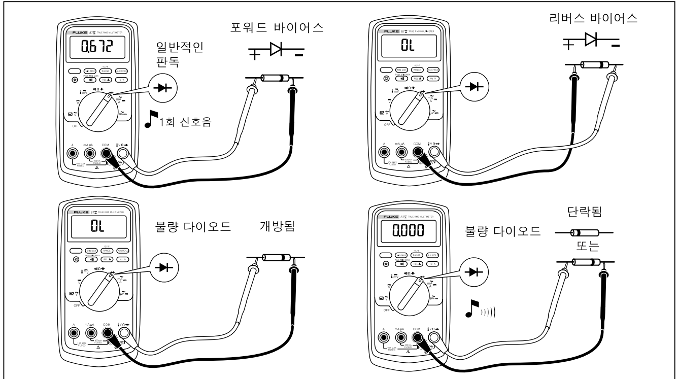
그림 7. 다이오드 테스트
