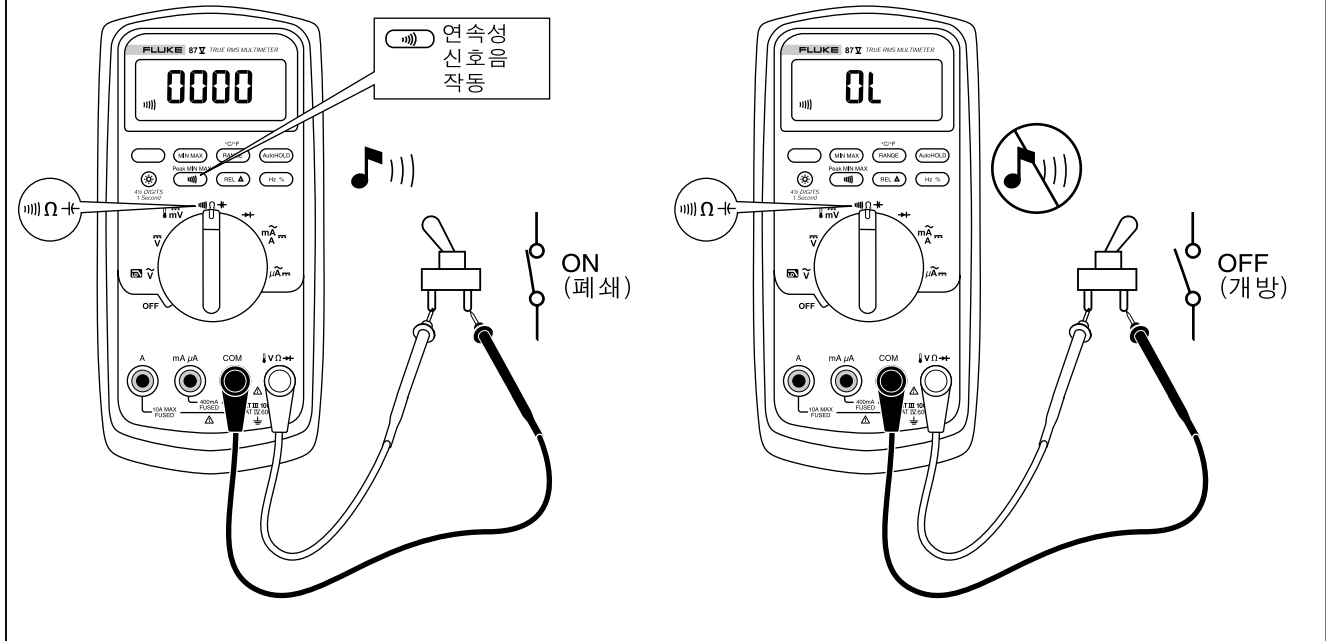
그림 4. 연속성 테스트
