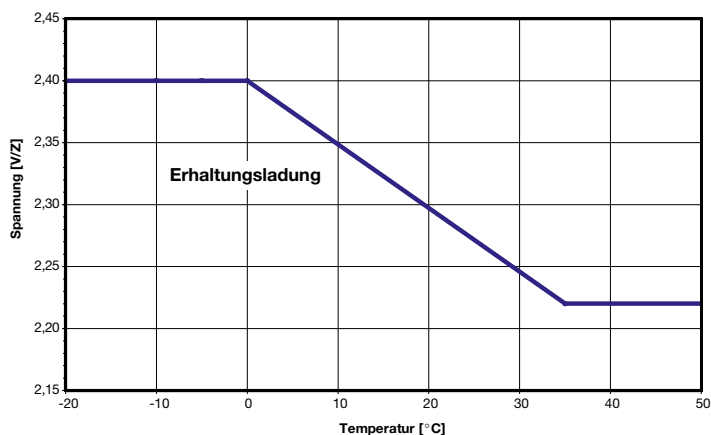
Bild 2: Marathon M/M-FT, Sprinter P/XP/FT, Sprinter S; Ladespannung über der Temperatur
