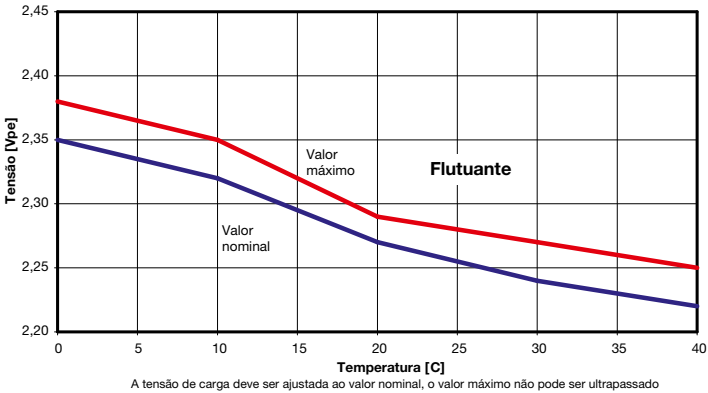
Fig.1: Marathon L/XL e Powerfit S; Tensão de carga vs. Temperatura
