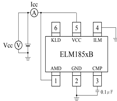
I cc 消費電流測定回路
