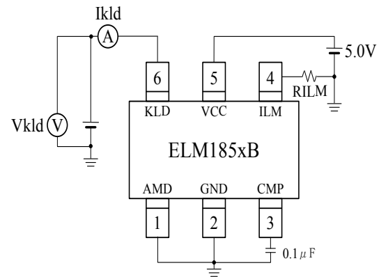
I kld 定電流測定回路
