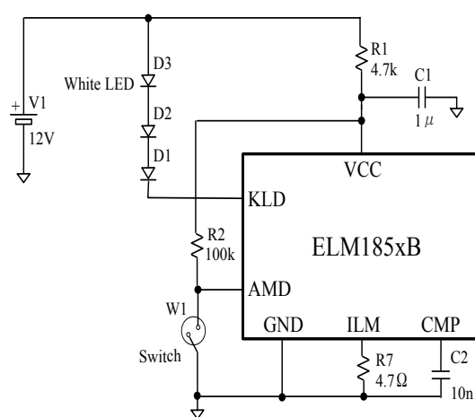
応用回路図 (6)
