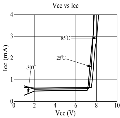
電源電圧対消費電流特性
