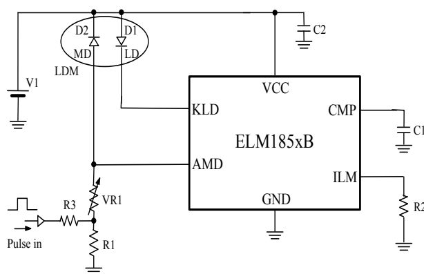
応用回路図 (4)
