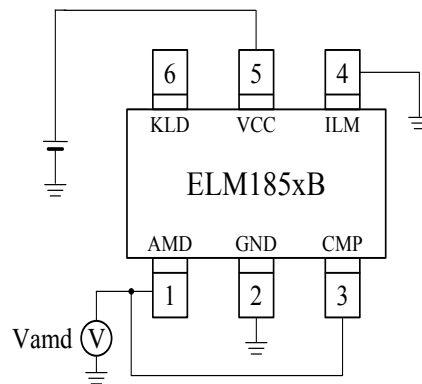
V amd 基準電圧測定回路
