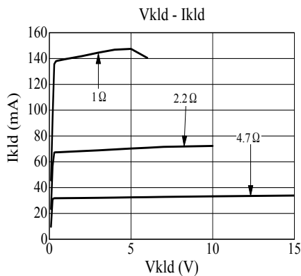
KLD 出力電流電圧特性
