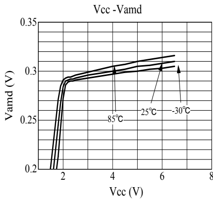
電源電圧対 AMD 基準電圧特性
