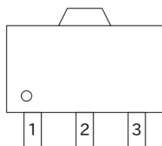
SOT-89(TOP VIEW)
