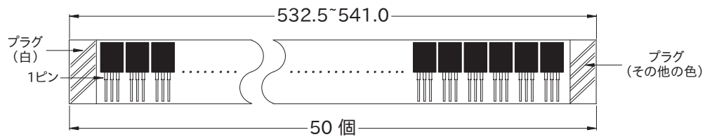
断面図
