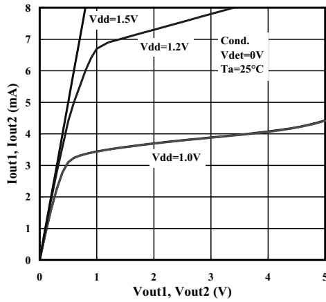
Iout-Vout
