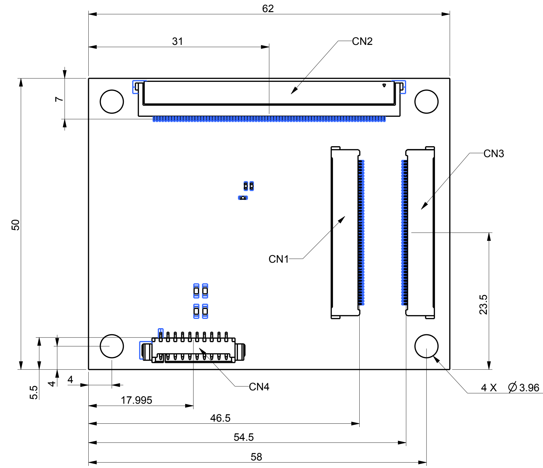
SCALE 0.100
