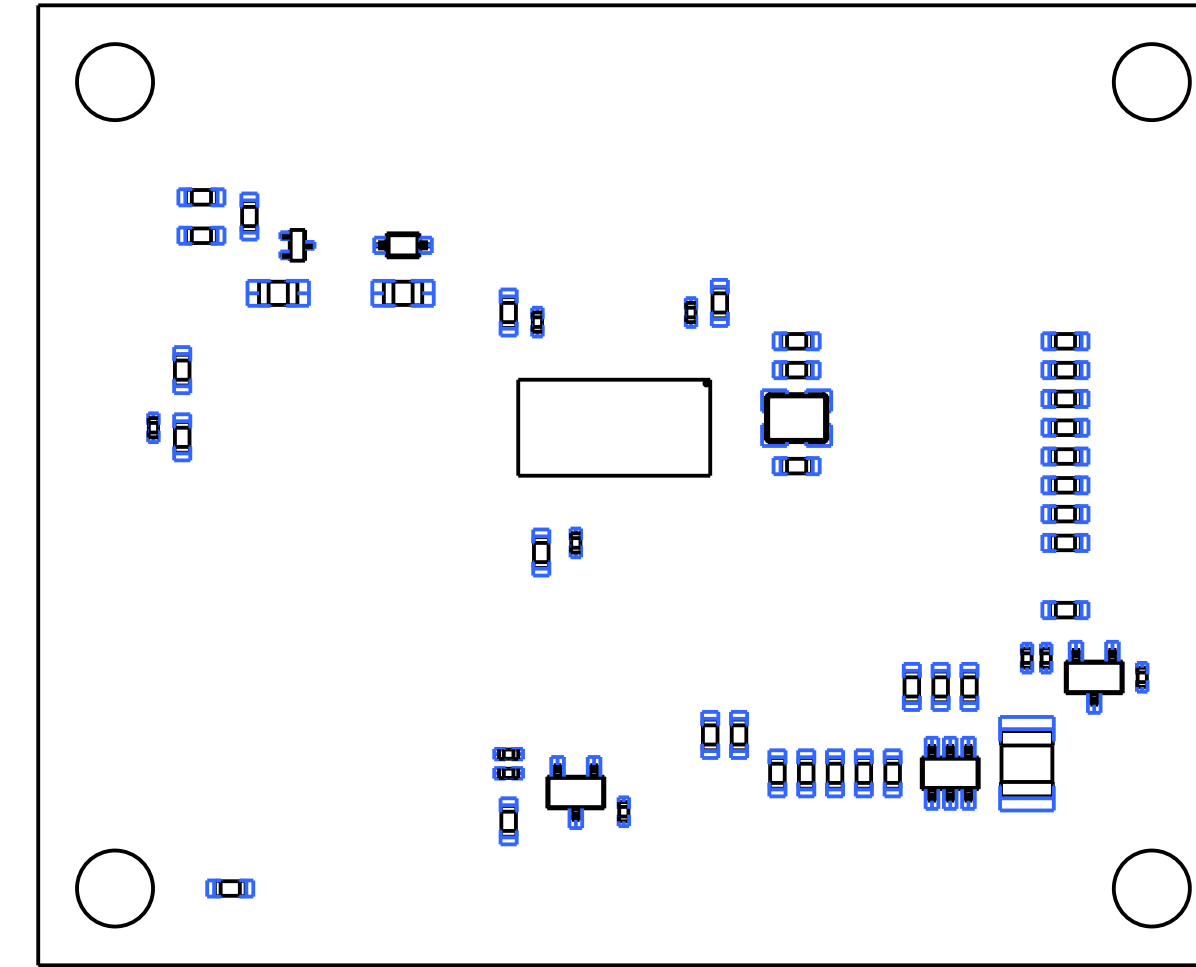
SCALE 0.100
