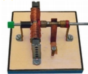
C-6145 Kit motor eléctrico básico.
