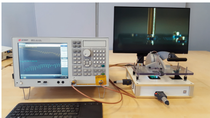
RF测试站
