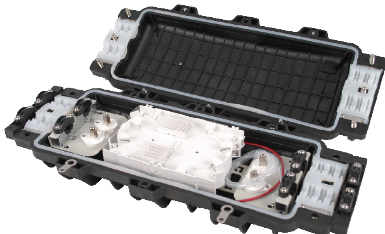
Models: F1-OSPDBC24 - 24 fiber F1-OSPDBC48 - 48 fiber
