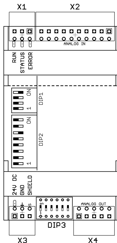
Ansicht von oben (Deckel geöffnet) (DIP1 und DIP2 im Gehäuse, DIP3 von außen zugänglich)
