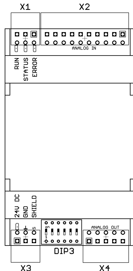
Ansicht von oben
