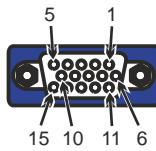
VGA
