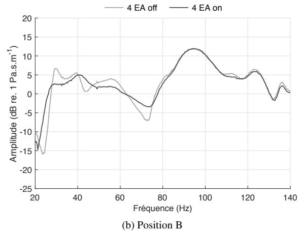
FIGURE 5 – Fonctions de transfert mesurées entre la vitesse de la membrane de la source sonore et le niveau de pression acoustique pour deux positions différentes dans la salle.
