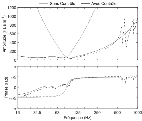
FIGURE 4 – Réponses en fréquence de l’impédance acoustique spécifique de l’absorbeur électroacoustique simulées (lignes continues) et mesurées (lignes pointillées) à l’extrémité d’un tube d’impédance avec et sans contrôle.
