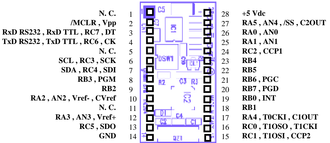
FIGURA 3: ZOCCOLO CON SEGNALI DEL MINI MODULO
