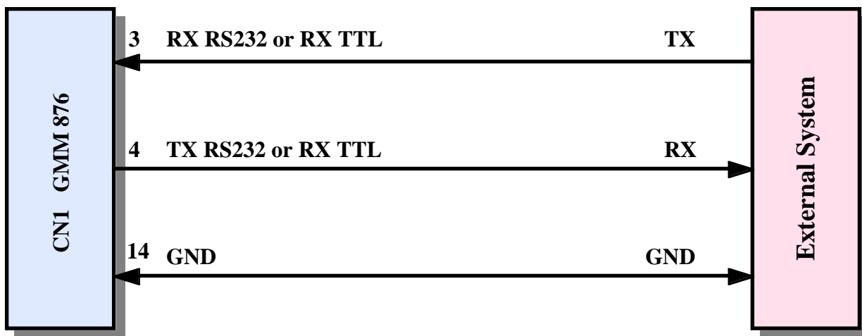
FIGURA 30: ESEMPIO COLLEGAMENTO SERIALE TTL
