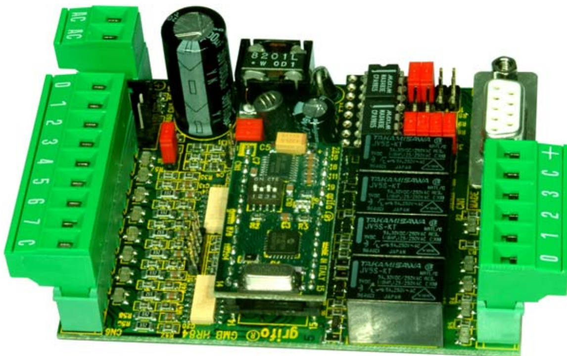
FIGURA 9: VISTA MODULO GMB HR 84 APERTO CON MONTATO UN GMM 876
