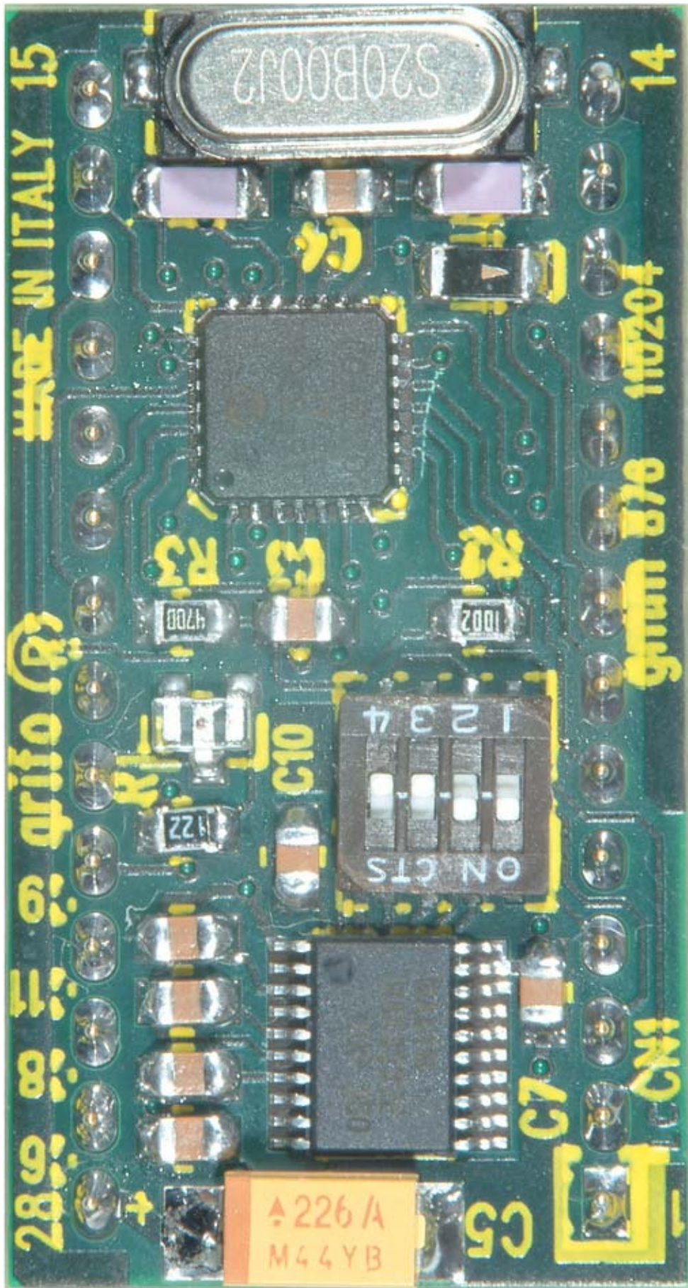
FIGURA 31: VISTA DALL'ALTO DEL MINI MODULO GMM 876
