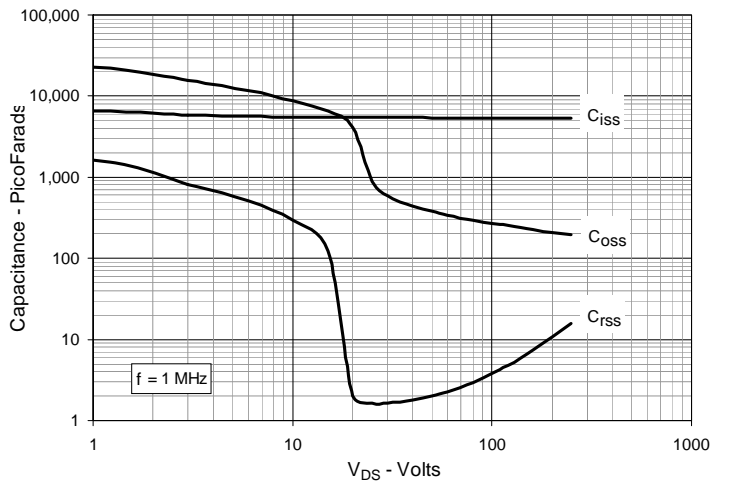
Fig. 12. Capacitance
