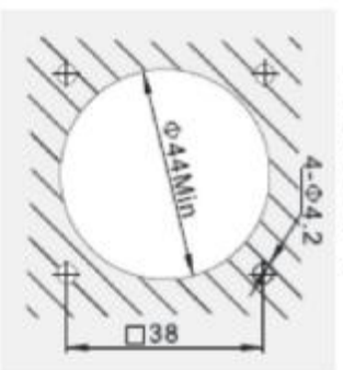
安装孔尺寸
