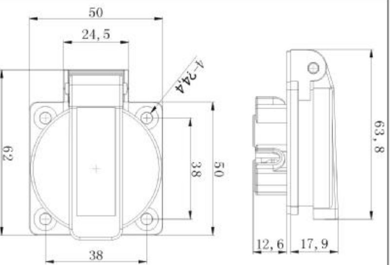
安装孔尺寸
