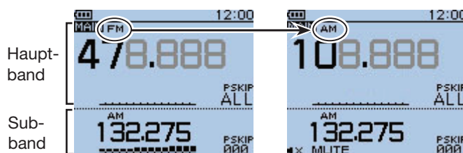
Wenn der Suchlauf im Hauptband das Flugfunkband scannt, ist die Subband-NF-Wiedergabe stummgeschaltet.
