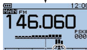
Wenn man das Sweepen gestoppt hat, kann man den Sweep-Marker mit [DIAL] auf das gewünschte Signal bewegen und dieses, je nach Voreinstellung, auch hören.
