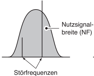
Auto-Notch-Filter ausgeschaltet
