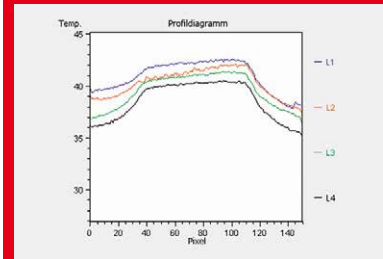
Temperaturprofil der definierten Linien L1-L4
