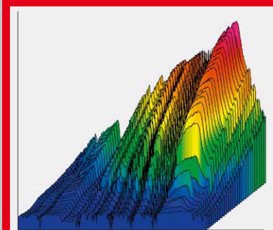
3D-Darstellung des Temperaturprofils der Linie L1 über die Zeit
