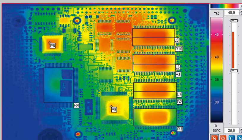
Thermogramm einer Leiterplatte mit Messdefinition
