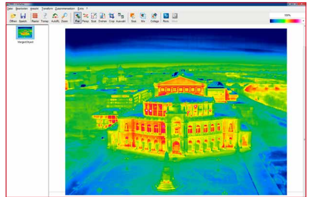
Automatisch zusammengefügtes Thermogramm
