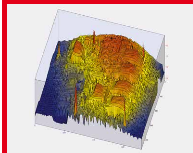
3D-Darstellung des Thermogramms
