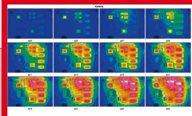
Galerieansicht der aufgenommenen Sequenz
