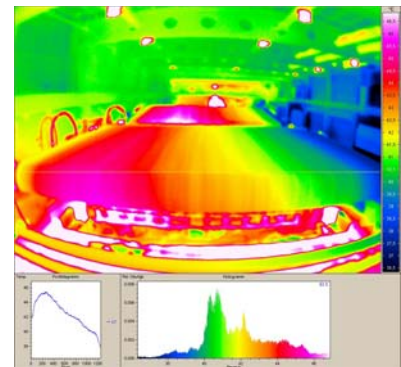
Abb. 1: Pressfilz mit Temperaturprofil
