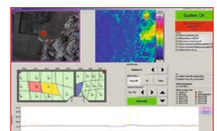
Mehrkamerasystem
