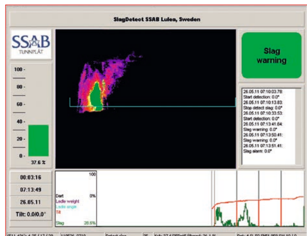
Prüf- und Überwachungssysteme zur Schlackedetektion
