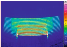
Heckscheibenheizung
