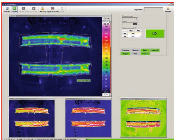
INDU-SCAN-Pressenüberwachung
