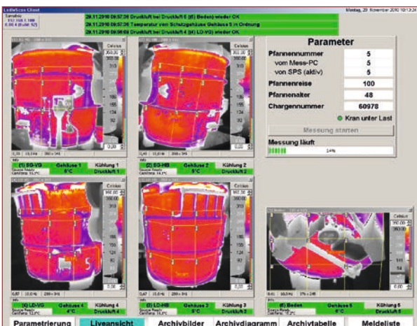
5-Seiten-Überwachung einer Pfanne mittels Mehrkopflösung
