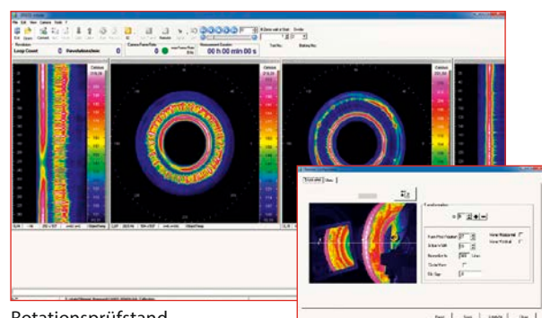
Rotationsprüfstand
