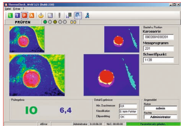
Automatische Schweißpunktprüfung
