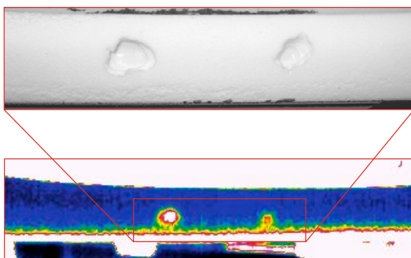
IR-Prüfbild
