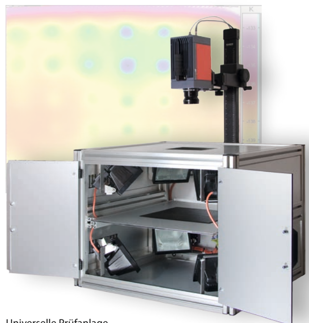
Universelle Prüfanlage
