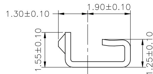
SEC:D-D
