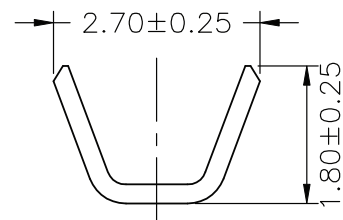
SEC:A-A
