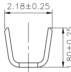
SEC:B-B
