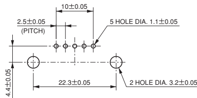
基板取付穴寸法(参考・装着面)
