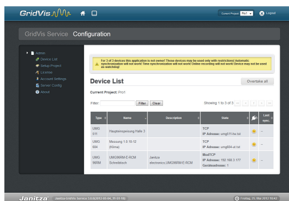
Рис. Системная версия GridVis (список устройств с сообщением об управлении)
