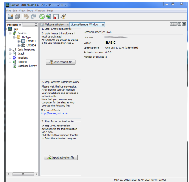
Рис. Окно диспетчера лицензий GridVis
