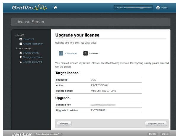
Рис. Сервер лицензирования GridVis (обзор лицензии)
