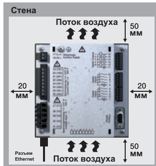
Или. Дополнительные данные по установке UMG508; вид сзади.
