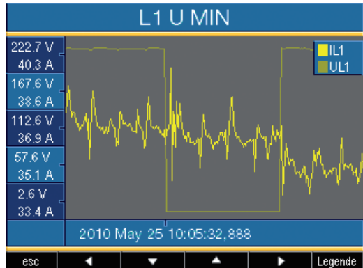
Иллюстрация отображения действующих значений за полный период для события.
