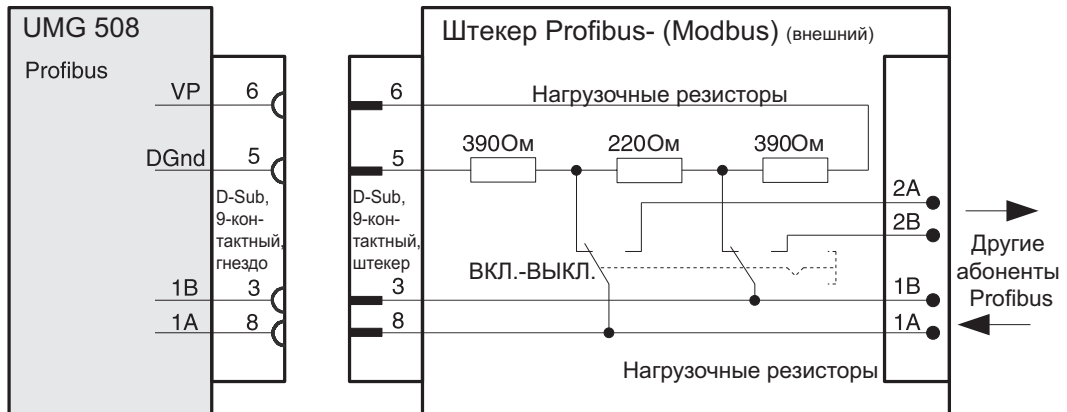
Иллюстрация. Штекерный разъем Profibus с согласующими резисторами.
