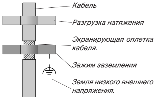
Иллюстрация. Схема экранирования в точке входа в шкаф.
