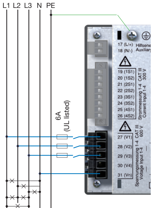
Иллю. Пример соединения для измерения напряжения.
