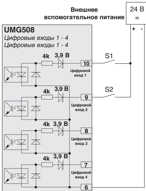
Иллю. Пример подключения внешних контактов S1 и S2 к цифровым входам 1 и 2.
