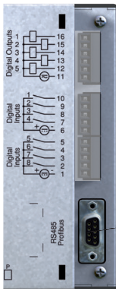
Илл. UMG508 с разъемом DSUB для интерфейса RS485.
