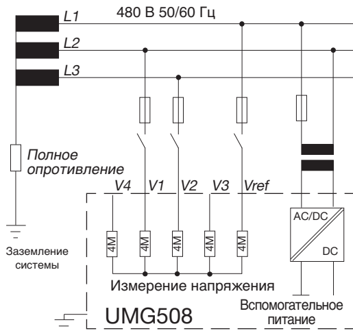
Иллюстрация. Главная принципиальная схема, UMG508 в сети IT без нейтрали (N).
