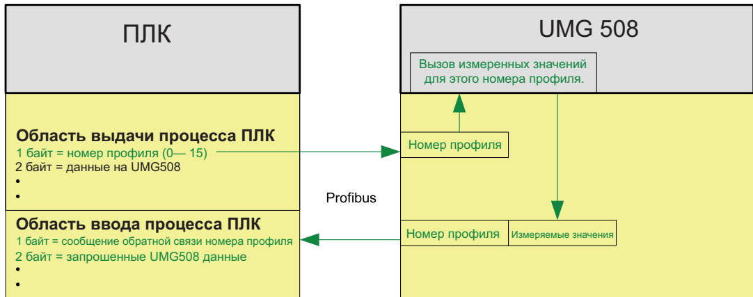
Илл. Блок-схема коммутации для обмена данными между ПЛК и UMG508.
