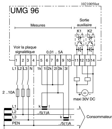
Fig.: Exemple de raccordement 2 Mesure 4 fils avec deux transformateurs d'intensité.
