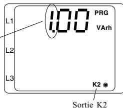
Fig. Utilisation comme sortie d'impulsions sur optocoupler
