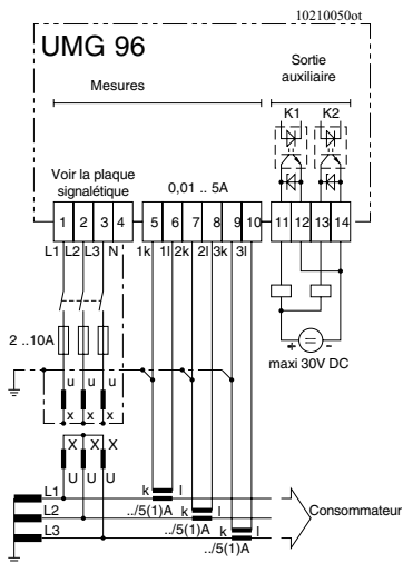
Fig.: Exemple de raccordement 3 Mesure 3 fils avec transformateurs d'intensité et trois transformateurs d'intensité.
