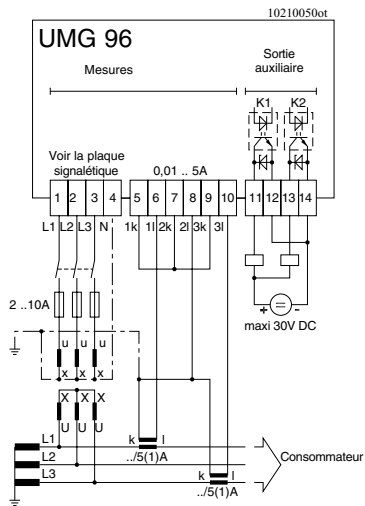
Fig.: Exemple de raccordement 4 Mesure 3 fils avec transformateurs d'intensité et deux transformateurs d'intensité.
