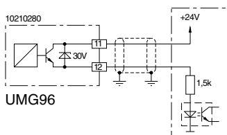
Fig. Utilisation comme sortie d'impulsions sur optocoupler
