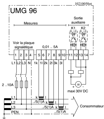
Fig.: Exemple de raccordement 1 Mesure 4 fils avec trois transformateurs d'intensité.
