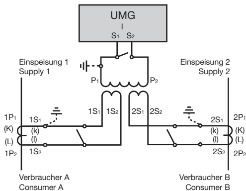
Abb. Strommessung über einen Summenstromwandler (Beispiel).
