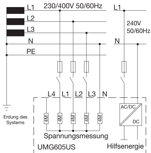
Abb.15.1 Prinzipschaltbild, UMG605US im TN-Netz.
