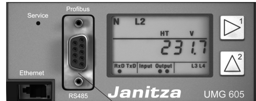
Abb.36.1 UMG605US mit Profibusschnittstelle.
