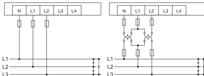
Abb.31.2 Anschlussbeispiele für die Spannungsmessung in „Dreiphasen-3-Leiternetzen“. (Anschlussvariante 1, siehe Seite 49)
