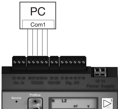
Abb.:33.1 Beispiel, ein UMG605US über die RS232 Schnittstelle mit einem PC verbinden.
