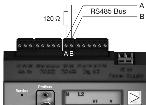
RS485-Schnittstelle, 2-poliger Steckkontakt mit Abschlusswiderstand (Art.-Nr. 52.00.008)
