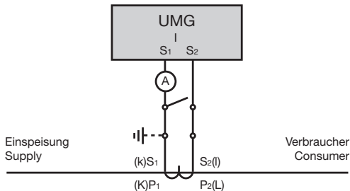
Abb.26.1 Beispiel, Strommessung über zusätzliches Amperemeter.
