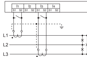
Abb.25.2 Strommessung, Anschlussbeispiel für die Anschlussvariante 0 (Siehe Seite 50).
