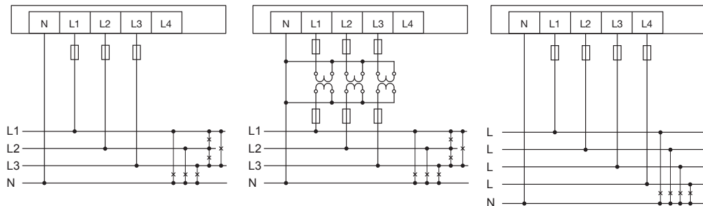
Abb.31.1 Anschlussbeispiele für die Spannungsmessung in „Dreiphasen-4-Leiternetzen“. (Anschlussvariante 0, siehe Seite 49)
