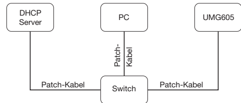
Abb. Anschlußbeispiel, UMG605US und PC bekommen die IP-Adresse von einem DHCP-Server automatisch zugewiesen.
