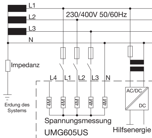
Abb.17.2 Prinzipschaltbild, UMG605US im IT-Netz mit N.
