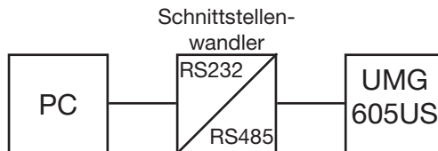
Abb.13.2 Anschluss eines UMG605US an einen PC über einen Schnittstellenwandler.
