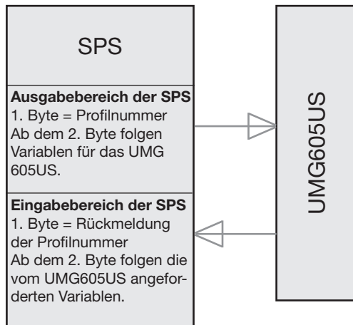
Abb.54.1 Blockschaltbild für den Datenaustausch zwischen SPS und UMG605US.
