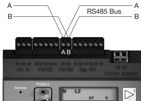
RS485-Schnittstelle, 2-poliger Steckkontakt
