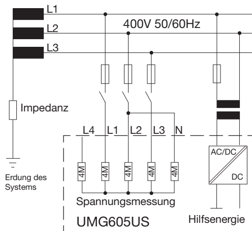
Abb.17.1 Prinzipschaltbild, UMG605US im IT-Netz ohne N.
