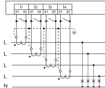
Abb.25.2 Strommessung, Anschlussbeispiel für die Anschlussvariante 0 (Siehe Seite 50).
