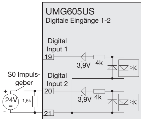
Abb.40.2 UMG605US mit Eingängen für 24V. Beispiel für den Anschluss eines S0 Impulsgebers an den digitalen Eingang 2.
