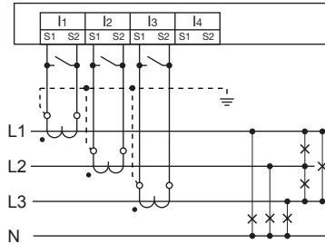
Abb.25.1 Strommessung, Anschlussbeispiel für die Anschlussvariante 0 (Siehe Seite 50).
