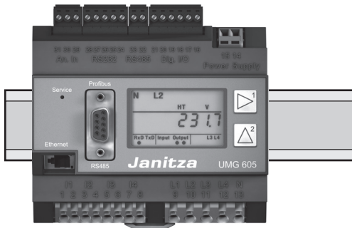
Abb.22.1 UMG605US auf Tragschiene nach DIN EN 60715.
