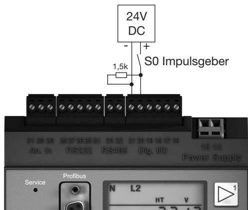
Abb.41.1 UMG605US mit Eingängen für 24V. Beispiel mit S0 Impulsgeber.
