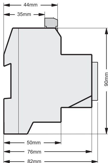
Seitenansicht
