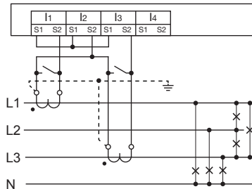
Abb.25.3 Strommessung, Anschlussbeispiel für die Anschlussvariante 0 (Siehe Seite 50).
