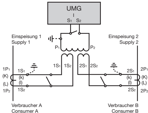
Abb.27.1 Beispiel, Strommessung über Summenstromwandler.
