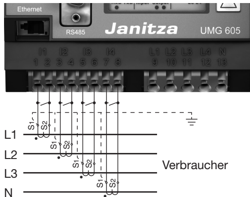
Abb.24.1 Anschlussbeispiel, Strommessung über Stromwandler.
