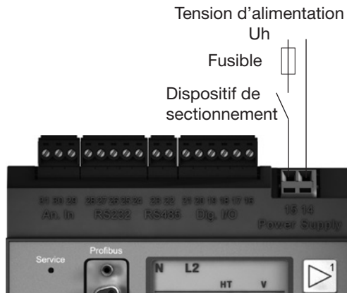
Fig. 23.1 Exemple de raccordement de la tension d'alimentation U_h .
