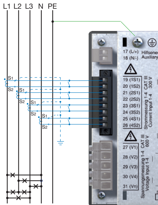
Afb. aansluitvoorbeeld, stroommeting via stroomtransformatoren.
