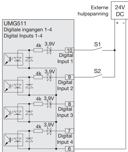
Afb. voorbeeld voor de aansluiting van de externe contacten S1 en S2 aan de digitale ingangen 1 en 2.
