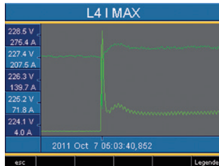
Afb. weergave van de effectieve waarden halve golf bij een voorval.
