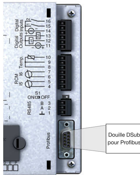
Fig. UMG 512 avec douille DSub pour Profibus (Vue de l'arrière).
