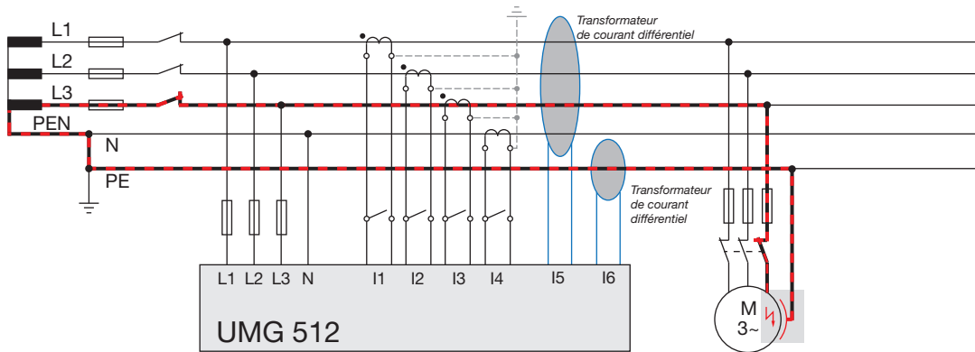
Fig. Exemple d'UMG 512 avec surveillance de courant différentiel par les entrées de mesure I5/I6.
