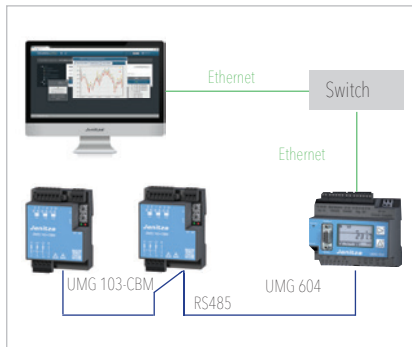
Anschluss mehrerer UMG 103-CBM an einen PC über ein UMG 604 (mit der Option Ethernet)
