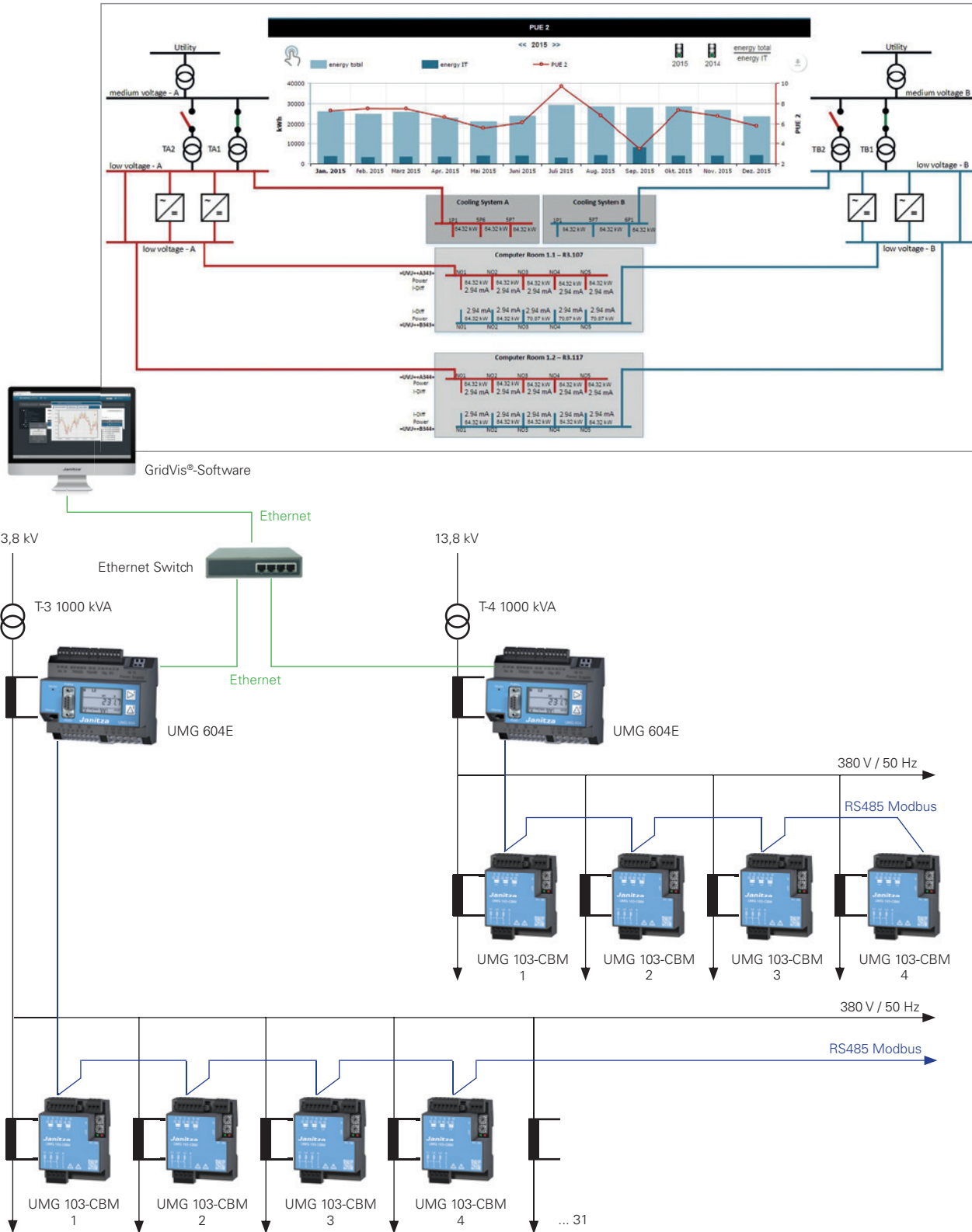
Abb.: Typische Applikationsabbildung mit 2 Einspeisungen, UMG 604 als Master-Messgeräte in der Haupteinspeisung und UMG 103-CBM zur Messung der Niederspannungsabgänge.
