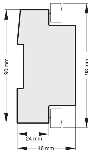
Seitenansicht
