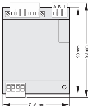
Vorderansicht
