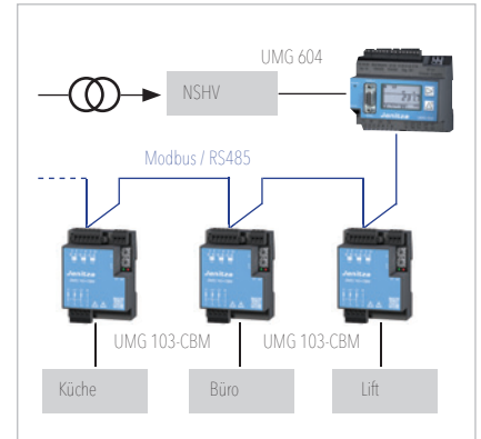
Topologiebeispiel UMG 604 (Master) – UMG 103-CBM (Slave)
