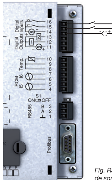
Fig. Exemple pour le raccordement des contacts de commutation externes S1 et S2 aux entrées numériques 1 et 2.
