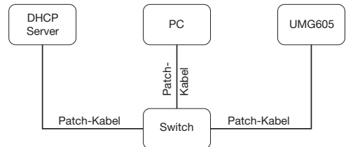
Abb. Anschlußbeispiel, UMG605 und PC bekommen die IP-Adresse von einem DHCP-Server automatisch zugewiesen.
