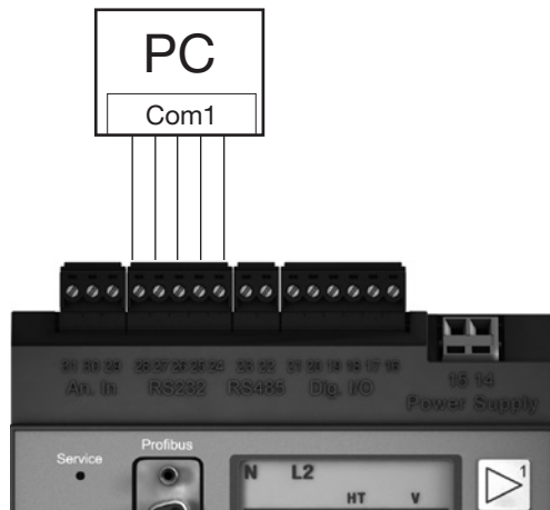
Abb.:33.1 Beispiel, ein UMG605 über die RS232 Schnittstelle mit einem PC verbinden.
