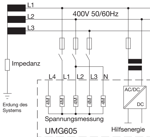
Abb. Prinzipschaltbild, UMG605 im IT-Netz ohne N.
