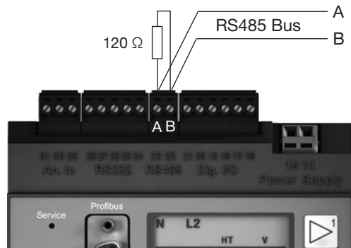
RS485-Schnittstelle, 2-poliger Steckkontakt mit Abschlusswiderstand (Art.-Nr. 52.00.008)
