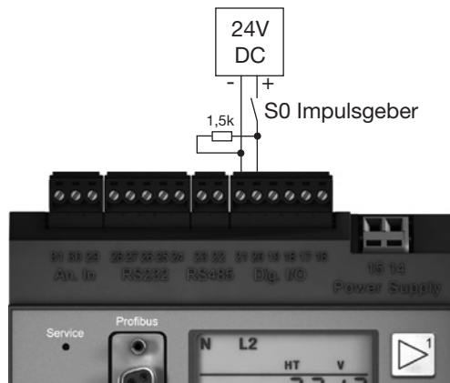
Abb.41.1 UMG605 mit Eingängen für 24V. Beispiel mit S0 Impulsgeber.
