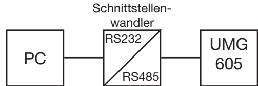
Abb. 13.2 Anschluss eines UMG605 an einen PC über einen Schnittstellenwandler.
