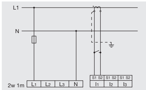
Abb. Messung einer Phase in einem Dreipha- sen-4-Leiternetz.
