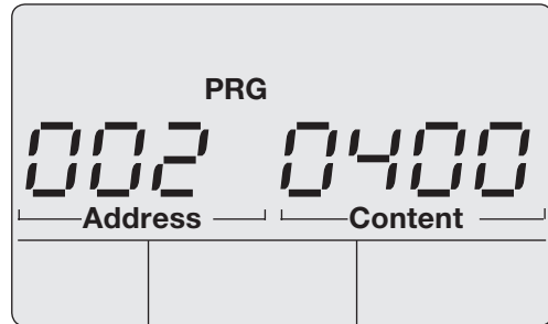
Abb. Beispiel; Spannungswandler (primär) für die Hauptmessung, Adresse 002 mit dem Inhalt „400“.
