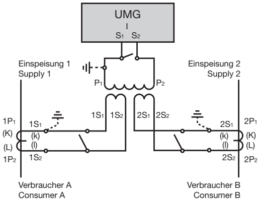
Abb. Beispiel, Strommessung über Summenstromwandler.
