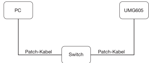
Abb. Anschlußbeispiel, UMG605 und PC benötigen eine feste IP-Adresse.
