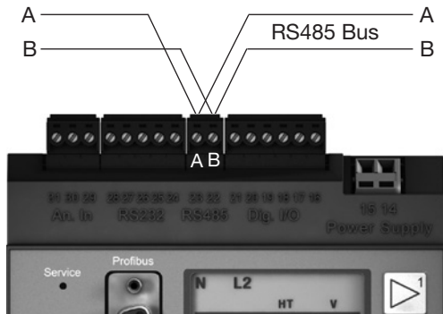
RS485-Schnittstelle, 2-poliger Steckkontakt
