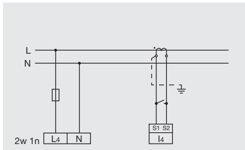
Abb. Messung mit einem Stromwandler.
