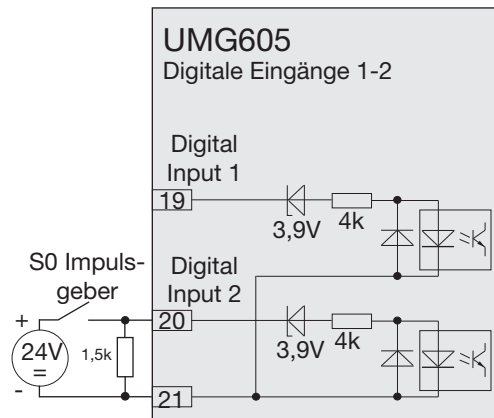
Abb.40.2 UMG605 mit Eingängen für 24V. Beispiel für den Anschluss eines S0 Impulsgebers an den digitalen Eingang 2.
