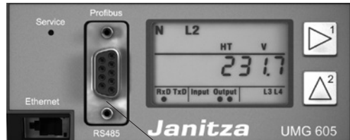
Abb.36.1 UMG605 mit Profibusschnittstelle.
