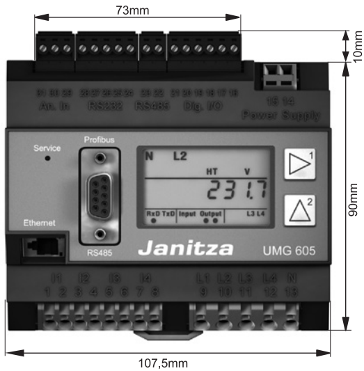
Vorderansicht
