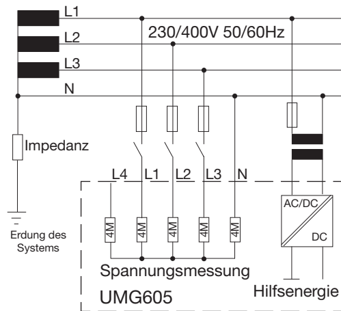
Abb. Prinzipschaltbild, UMG605 im IT-Netz mit N.
