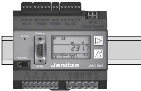
Abb.22.1 UMG605 auf Tragschiene nach DIN EN 60715.
