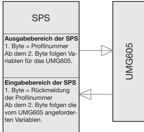
Abb.54.1 Blockschaltbild für den Datenaustausch zwischen SPS und UMG605.
