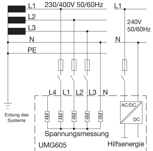
Abb. Prinzipschaltbild, UMG605 im TN -Netz.
