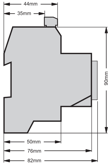
Seitenansicht
