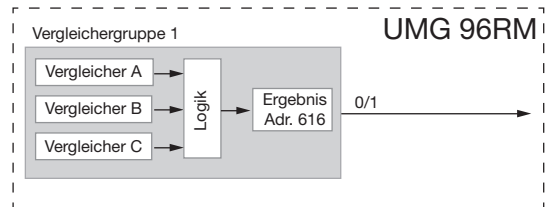
Blockschaltbild: Verwendung der Vergleichergruppe 1
