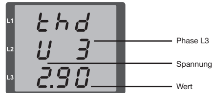
Abb. Anzeige des Oberschwingungsgehalt THD der Spannung aus der Phase L3 (Beispiel).
