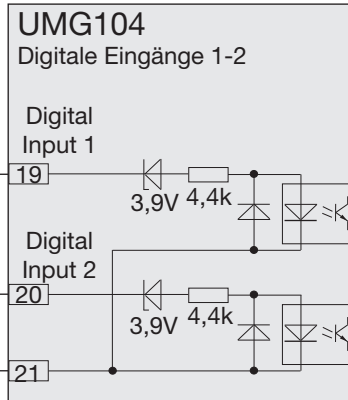
Abb.40.2 Beispiel für den Anschluss der externen Schaltkontakte S1 und S2 an die digitalen Eingänge 1 und 2.
