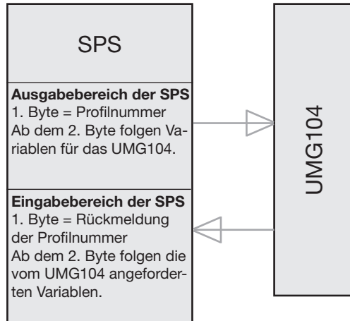
Abb.54.1 Blockschaubild für den Datenaustausch zwischen SPS und UMG104.
