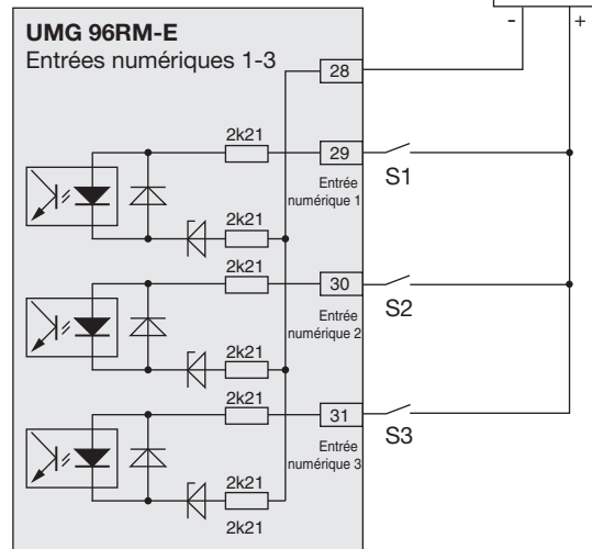
Fig. Exemple pour le raccordement des contacts de commutation externes S1 et S2.
