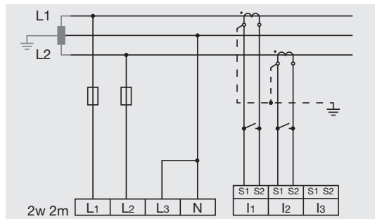
Рис. Измерение в однофазной 3-проводной сети. I_2 и I_3 не рассчитываются и устанавливаются равными нулю.
