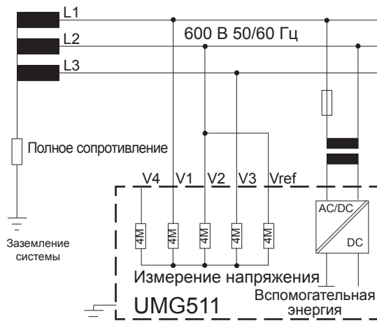
Рис. Принципиальная схема, UMG511 в IT-сети без N.
