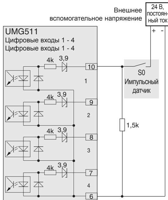
Рис. Пример подключения импульсного S0-датчика на цифровой вход 1.
