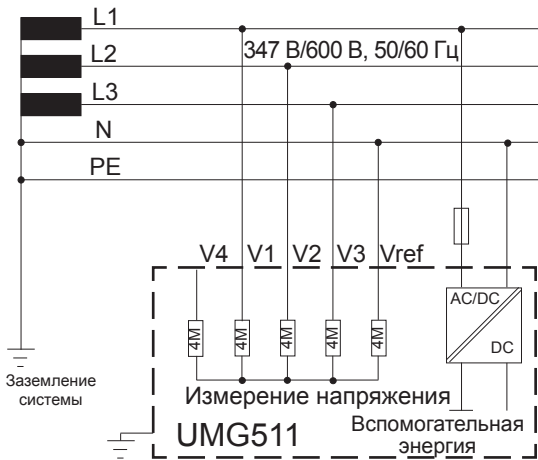
Рис. Принципиальная схема, UMG511 в TN-сети.
