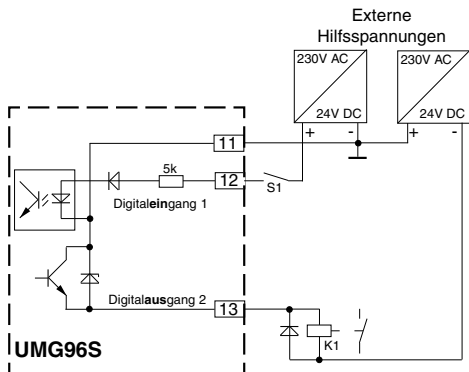
Abb.: Anschlussbeispiel für einen Digitaleingang und einen Digitalausgang.
