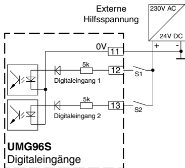
Abb.: Anschlussbeispiel für die Digitaleingänge.
