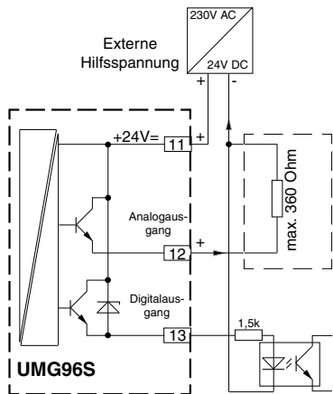
Anschlussbeispiel: UMG96S mit einem Analogausgang und einem Digitalausgang.
