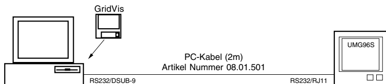
Abb. Das UMG96S mit einem PC über ein PC-Kabel verbinden.
