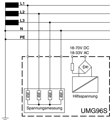
Abb. Blochschaubild Betriebsspannungsgewinnung und Messspannung.
