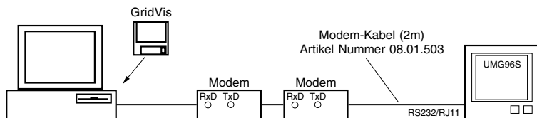
Abb. UMG96S über Modem mit einem PC Verbinden.
