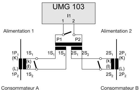
Fig.: Exemple de mesure d'intensité par un convertisseur de courant total.
