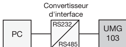
Fig. Raccordement d'un UMG103 par un PC par le biais d'un transformateur d'interface.
